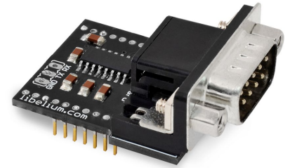
Figure: RS-232 Serial / Modbus module
