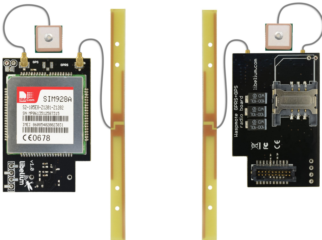
Figure: GPRS+GPS module
