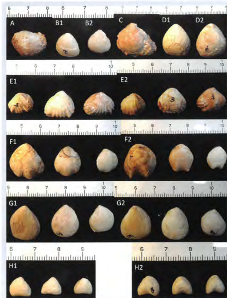
Abb. 5: Brachiopoden des Erlakogels. A Disperiferina sp. (Unter Lias) B ? Lobothyris sp. juv. (Mittel Lias); 1 (von unten), 2 (von oben fotografiert) C Liospiriferina aff. obtusa /OPPEL 1861 (Unter Lias) D Zeilleria mutabilis /OPPEL 1861 (Unter Lias); 1 (von oben), 2 (von unten fotografiert) E Gerippte Rhynchonellidae, wie Cuneirhynchia cartieri /OPPEL 1861 und ? Calcirhynchia plicatissima /QUENSTEDT 1852 (Unter Lias); 1 (von unten), 2 (von oben foto- graphiert) F „ Terebratula “ schlosseri /BÖSE 1897 (Mittel Lias); diese Art findet man nur am Erlakogel und in Kramsach/Tirol; 1 (von unten), 2 (von oben fotografiert) G „ Terebratula “ glacilicostata /BÖSE 1897 (Mittel Lias); 1 (von unten), 2 (von oben fotografiert) H Zeilleria aff. thurwieseri /BÖSE 1897 (Mittel Lias); 1 (von unten), 2 (von oben fotografiert)
