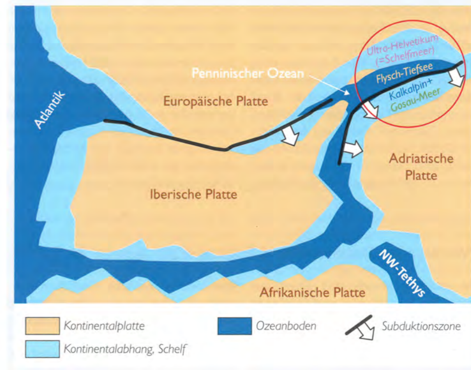
Abb. 9: Der Penninische Ozean stellte eine Verlängerung des Nordatlantiks nach Osten zur Tethys dar. Diese schematische, paläogeografische Karte der nordwestlichen Tethys und ihrer angrenzenden Gebiete zeigt rot umrandet die Position des „Ur-Traunsee-Ostufers“ im beginnenden Alt-Tertiär (vor ca. 65 Mill. Jahren). Zeichnung: Johannes Thomas Weidinger, Johannes Mattes
