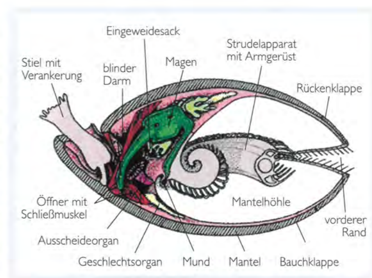
Abb. 4: Längsschnitt durch einen Brachiopoden. Zeichnung: Plöschinger & Karanitsch (2002)
